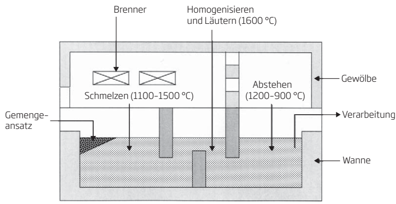
Abb. 6.1: Glasschmelzwanne (nach [2])
