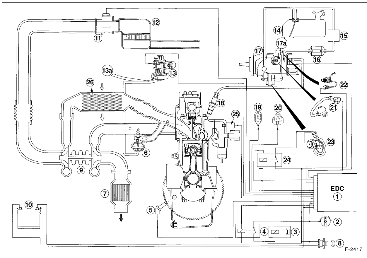
Schemazeichnung Diesel-Einspritzanlage
