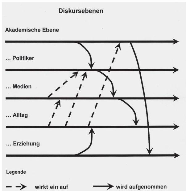
Abb. 6: Diskursebenen
