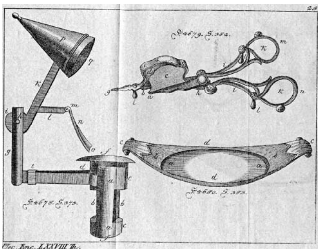
Abbildung 1: Lichtschere. Illustration des entsprechenden Eintrags im 1800 erschienenen 78. Band der maßgeblich von Johann Georg Krünitz verantworteten Oeconomischen Encyclopädie , deren 272 Bände zwischen 1773 und 1858 veröffentlicht wurden.
