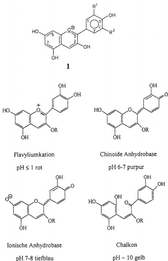
Abb. 4 Die pH-abhängigen Grundstrukturen der Anthocyane. (Aus: G. Schwedt, Experimente mit Supermarktprodukten , Wiley-VCH, Weinheim, 3. Aufl. 2009.)
