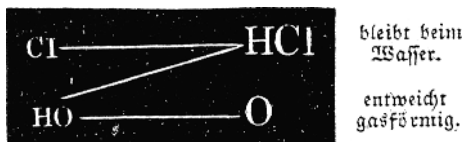
Abb. 2 Stöckhardts Darstellung der Reaktion zwischen Chlor und Wasser als Wahlverwandtschaft . (Aus: A. Stöckhardt, Die Schule der Chemie , »Chlorgas und Chlorwasser«, S. 155, 10. Aufl. 1858.)
