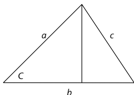
Abbildung 6: Unterteilung eines Dreiecks in zwei rechtwinklige Dreiecke.
