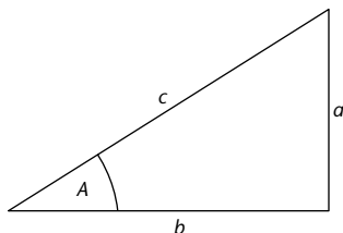
Abbildung 5: Trigonometrie basiert auf einem rechtwinkligen Dreieck.
