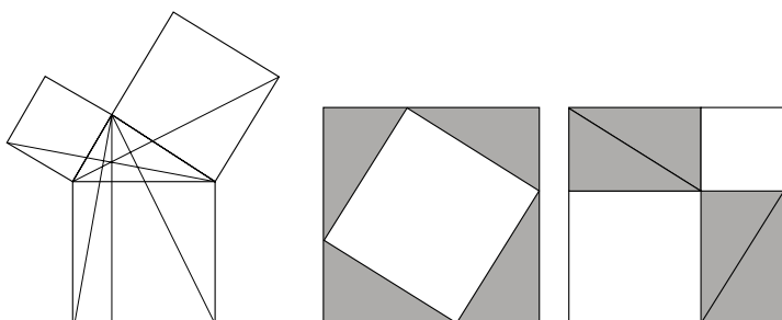
Abbildung 2: Links: Konstruktionsgeraden für Euklids Beweis des Satzes des Pythagoras. Mitte und rechts: Alternativer Beweis für den Satz. Die äußeren Quadrate haben die gleiche Fläche, und alle schattierten Dreiecke haben ebenfalls die gleiche Fläche. Daher hat das gekippte weiße Quadrat die gleiche Fläche wie die beiden anderen weißen Quadrate zusammen.
