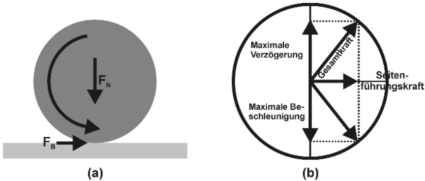
Abbildung 1.11: Die Reibungskraft bei einem Rad (a) und der kammförmige Reibkreis (b)
