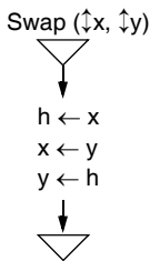
Abb. 1.9 Algorithmus Swap
