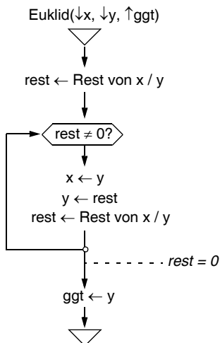
Abb. 1.12 Euklidischer Algorithmus
