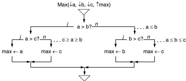
Abb. 1.10 Algorithmus Max
