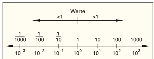
Bild 2: Zehnerpotenzen
