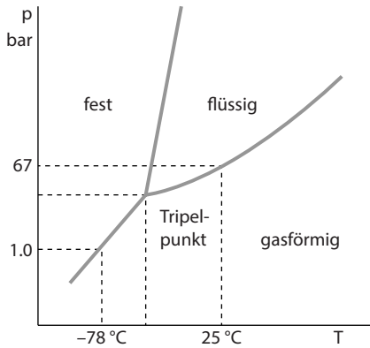
Abb. 1.1 Phasendiagramm von Kohlenstoffdioxid.
