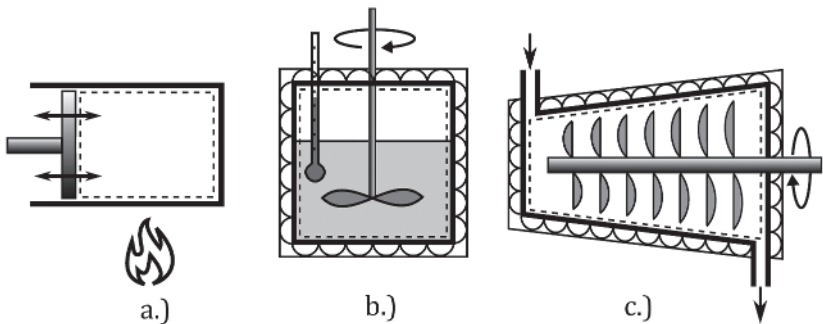
Abbildung 1.3 Beispiele verschiedener Systeme mit ihren Eigenschaften und gestrichelt dargestellten Systemgrenzen (alle Systeme übertragen Arbeit über ihre Grenzen): a.) verschieblicher Kolben mit beheiztem Zylinder (geschlossen, bewegliche Systemgrenze), b.) wärmeisolierter Rührbehälter (geschlossen, adiabatisch), c.) wärmeisolierte Dampfturbine (offen, adiabatisch).
