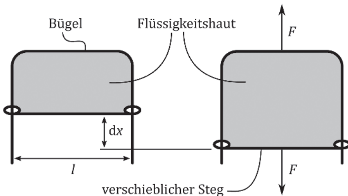
Abbildung 1.8 Einfache Messvorrichtung zur Bestimmung der Oberflächenspannung (Erklärung im Text).
