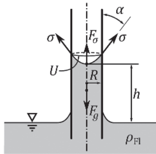
Abbildung 1.11 Kapillarwirkung mit dargestellten wirkenden Einzelkräften.
