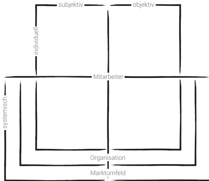
Abb. 1.2: Mitarbeiter-Organisation-Markt-Quadranten
