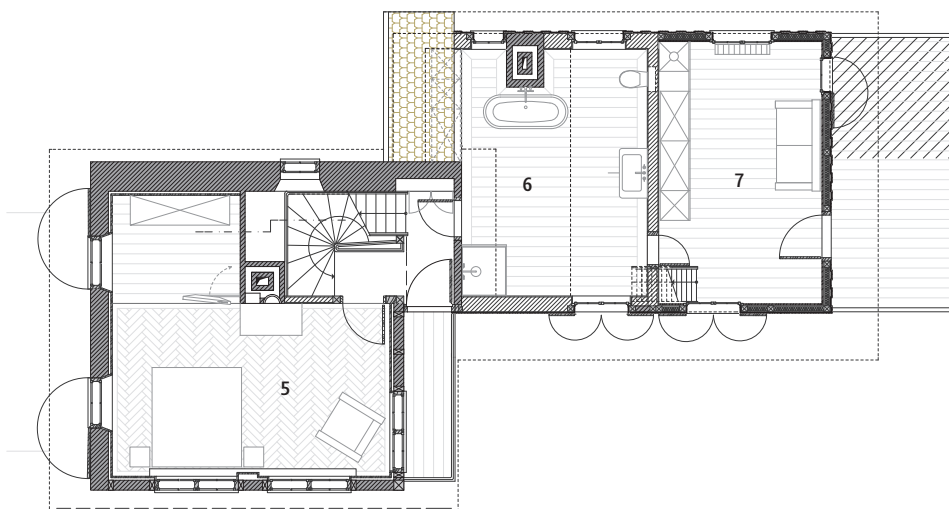
Obergeschoss
