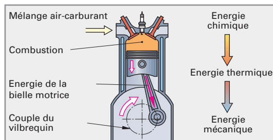
Illustration 2 : Conversion énergétique d'un moteur Otto
