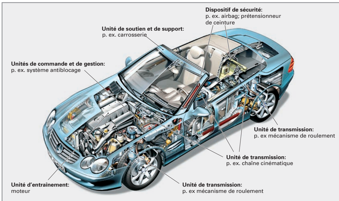
Illustration 1 : Le système véhicule à moteur et ses unités de fonction
