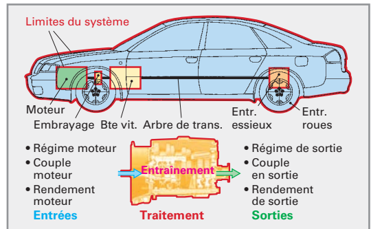
Illustration 3 : Sous-système : entraînement
