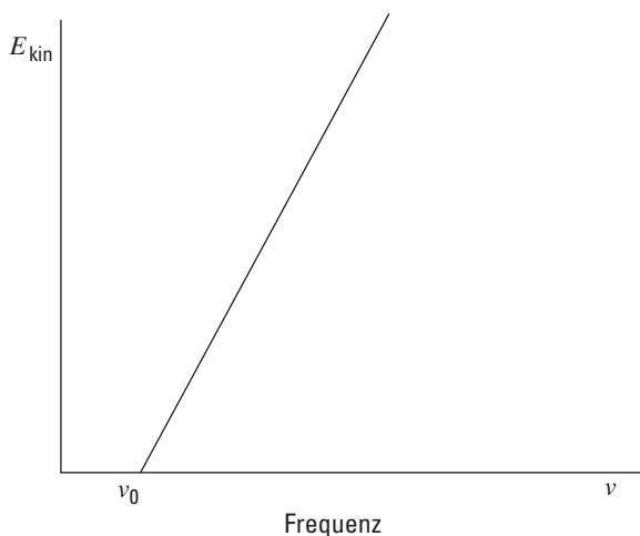
Abbildung 1.4: Kinetische Energie E_{\text{kin}} der emittierten Elektronen als Funktion der Frequenz \nu des einfallenden Lichts
