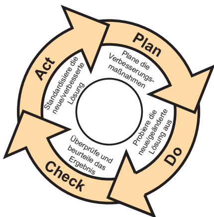
Bild 1: PDCA-Zyklus
