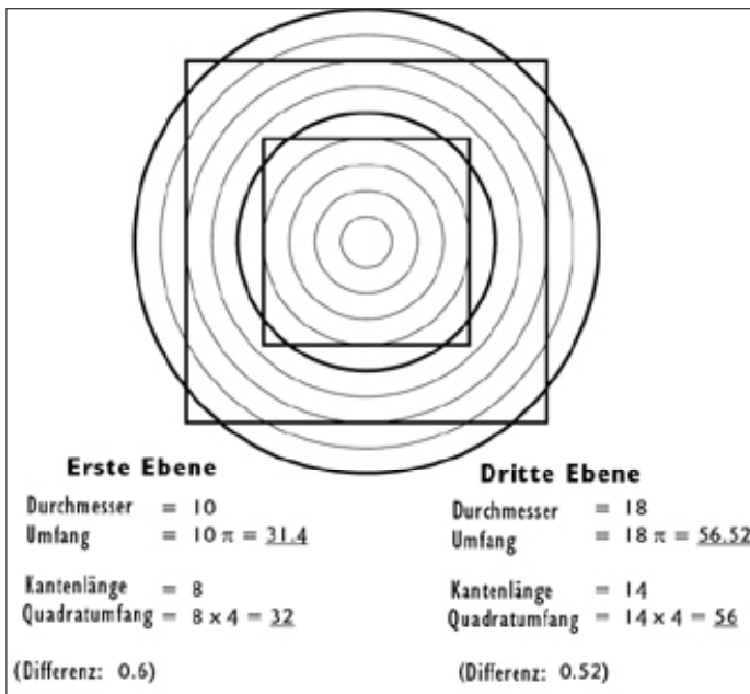
Abb. 9-2. Erste und dritte Ebene des menschlichen Bewusstseins; Verhältnis entspricht nahezu perfekt dem Phi-Quotienten.
