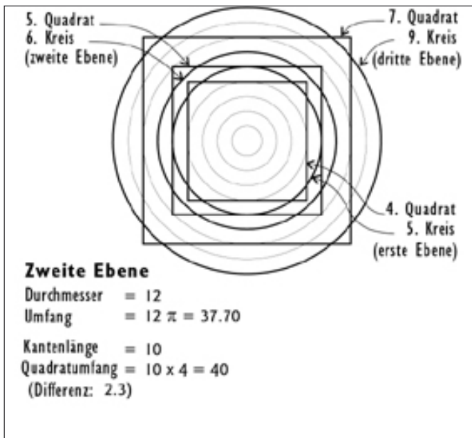
Abb. 9-3. Die drei geometrischen Ebenen des menschlichen Bewusstseins auf der Erde: Quadrat 4 und Kreis 5 = erste Ebene (Urvölker); Quadrat 5 und Kreis 6 = zweite (derzeitige) Ebene; und Quadrat 7 und Kreis 9 = dritte (Christus-) Ebene.
