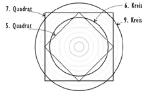
Abb. 9-4. Durch Drehung des zur zweiten Ebene gehörigen Quadrats um 45 Grad entsteht eine Brücke zwischen zweiter und dritter Bewusstseinsstufe.
