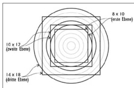
Abb. 9-5. Die drei Ebenen des menschlichen Bewusstseins als Einheiten oder Radien in ihren Kreis-Quadrat-Paaren.
