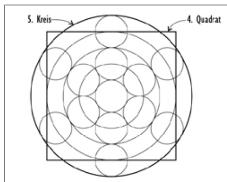
Abb. 9-6. Frucht des Lebens über erster Bewusstseinssebene.
