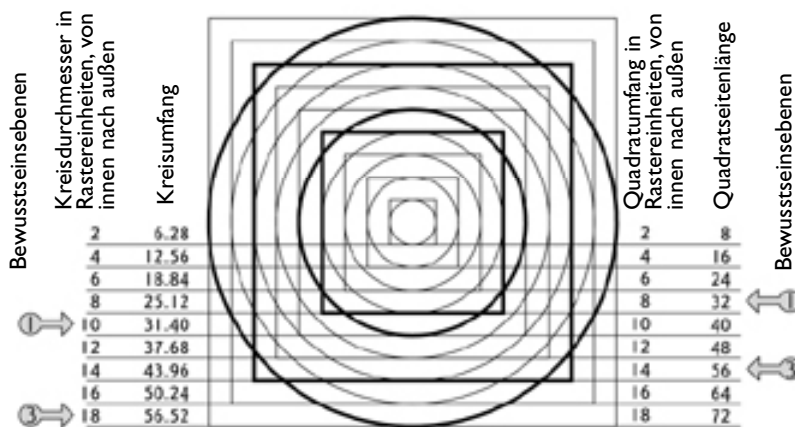
Abb. 9-1. Konzentrische Kreise und Quadrate. Die dickeren Kreise und Quadrate sind die Paare, die dem Phi-Quotienten nahekommen. Sie kennzeichnen ferner die Position der ersten und dritten Ebene des menschlichen Bewusstseins. (Eine Einheit im Raster entspricht einem Radius des Mittelkreises oder der Hälfte des umgebenden Quadrats. Man kann sehen, dass der Durchmesser des Mittelkreises der Länge einer Seite des Quadrats entspricht, das diesen Kreis umgibt.)
