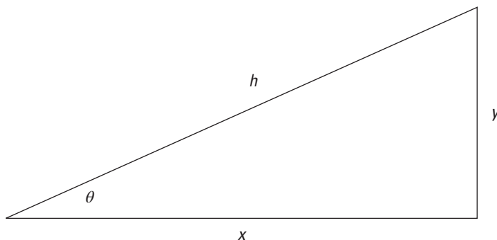
Abbildung 1.1: Ein Dreieck
