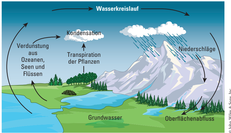
Abbildung 1.2: Der hydrologische Kreislauf
