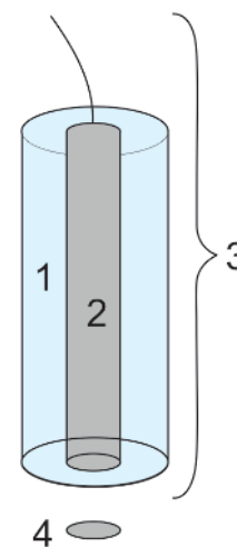
Abb. 1.2 Umgangssprachliche und elektrochemische Bedeutung des Begriffs „Elektrode“.
