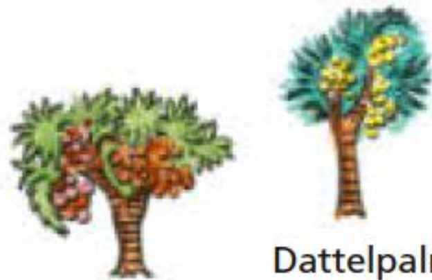
Feigenbaum
