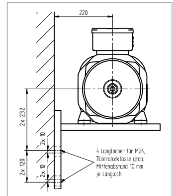
Bild 1: Maßskizze der Konsole
