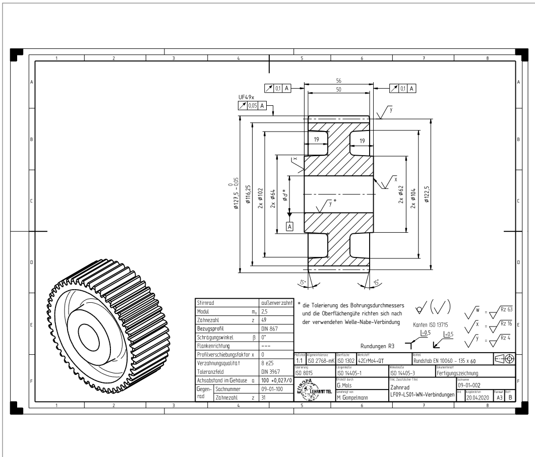
Bild 1: Zahnrad
