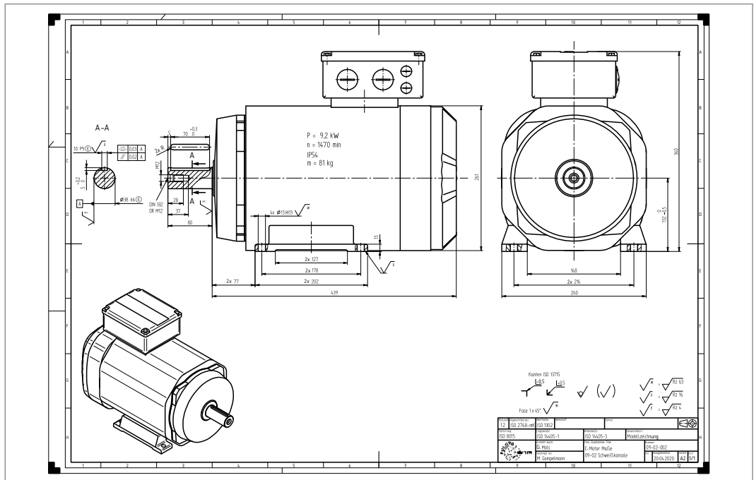
Bild 2: Maße des Elektromotors
