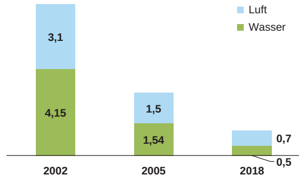
Abb. 1.1 Produktionsspezifische Umweltbelastung in kg je Tonne Verkaufsprodukt der BASF SE für 2002, 2005 und 2018.
