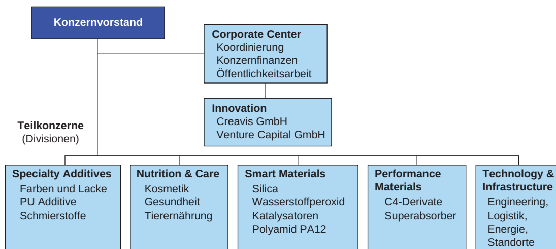
Abb. 1.3 Organisationsschema eines chemischen Großunternehmens am Beispiel der Evonik Industries AG (2022).
