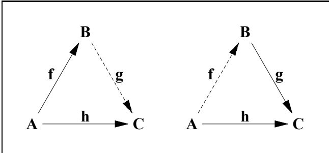
Kommutative Abbildungsdiagramme.
