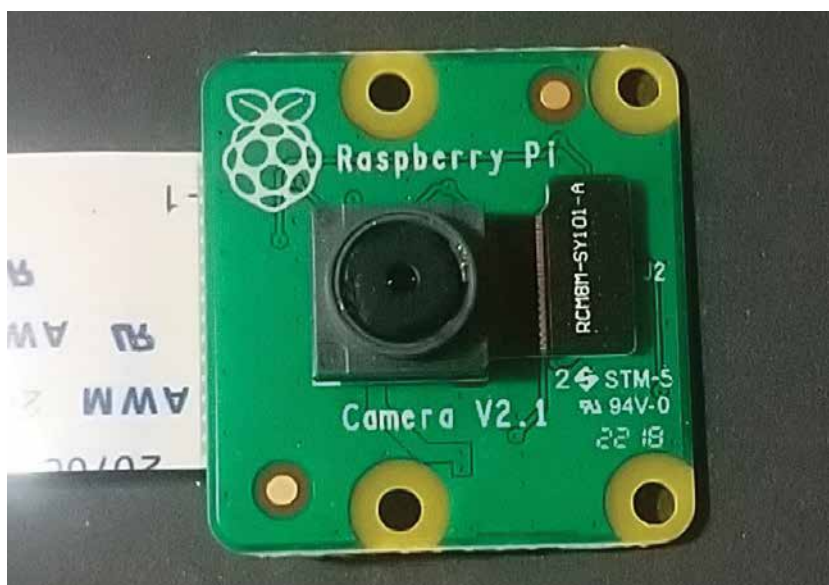
Abb. 9-1 Das Kameramodul des Raspberry Pi
