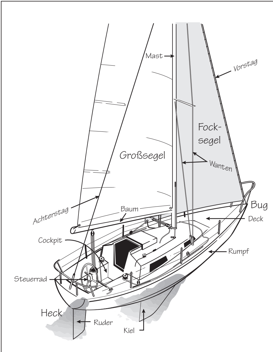
Abbildung 1.5: Die wesentlichen Teile eines Kiebootes.
