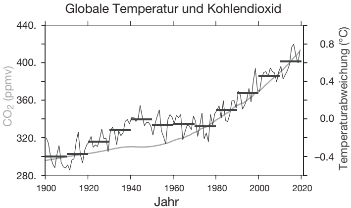
Abb. 1: Die global gemittelten jährlichen Werte der Temperatur an der Erdoberfläche als Abweichungen gegenüber dem Referenzzeitraum 1961–1990 und die Dekaden-Mittelwerte (schwarze Balken) zwischen 1900 und einschließlich 2019 sowie die jährlichen Werte der Konzentration von Kohlendioxid (CO 2 ) in der Luft (grau; ppm: parts per million, Teile pro eine Million).
