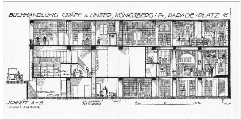
Schnitt, 1924.
