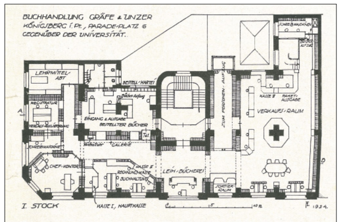
Grundriss 1. OG, 1924.
