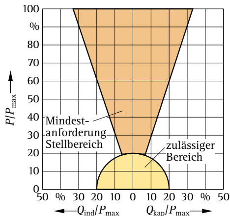
Bild 9.1 Geforderter Blindleistungsbereich von Erzeugungsanlagen mit \sum S_{E, \max} \leq 4,6 \text{ kVA} bei Wirkleistungseinspeisung im Niederspannungsnetz (nach Bild 5 [4.2])
