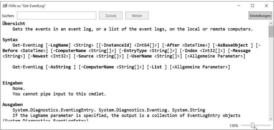
Abbildung 2.3: Hilfeinformationen zu einem Cmdlet abrufen.
