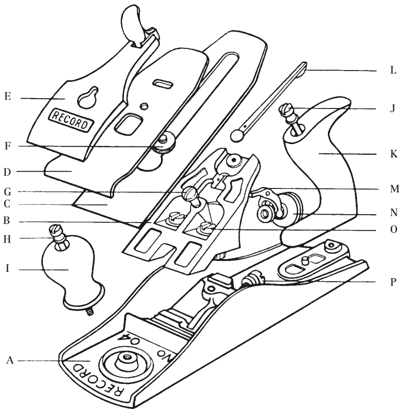
Abb. 1: Der Metallhobel und seine Einstellmechanismen A-Körper, B-Frosch, C-Eisen, D-Spanbrecher, E-Klappe, F-Spanbrecherschraube, G-Klappenschraube, H-Mutter und Schraube des Knopf, I-Knopf, Mutter und Schraube des Griffs, K-Griff, L-seitlicher Verstellhebel, M-Y-Verstellhebel, N-Eiseneinstellrad, O-Froschschauben, P-Froscheinstellschraube
