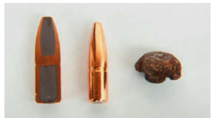
Swift-A-Frame (Zweikammer-Verbundgeschoss)
