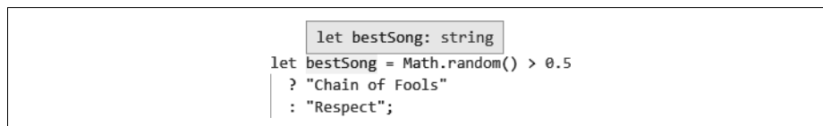
Abbildung 2-2: TypeScript meldet aufgrund einer Ableitung aus dem ternären Ausdruck, dass eine let -Variable den Literaltyp string hat.
