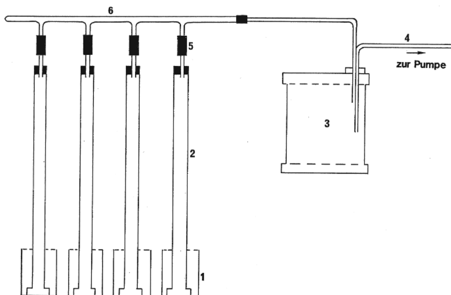
Abb. 1.1 Apparatur zur Technik der „fraktionierten Filtration“ mit mehreren Säulen für Petroleum nach der Methode von Day, um 1900. 1: Vorratsgefäße für Petroleumproben, 2: Säulen mit Adsorbentien, 3: Kammer zum Auffangen der Fraktionen, 4: Glasrohr zur Pumpe, 5 und 6: Verbindungssteile. Quelle: Schwedt (1982).
