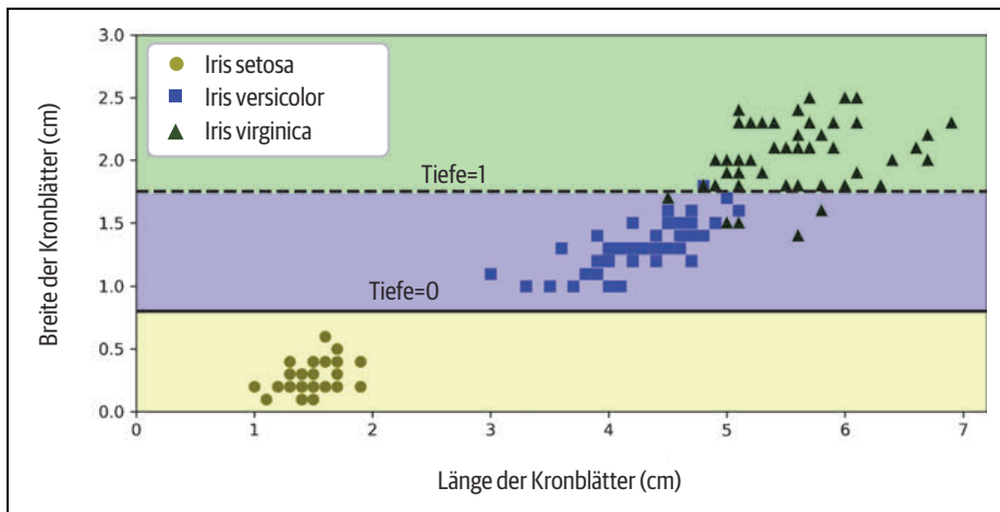
Abbildung 6-9: Ein erneutes Trainieren des gleichen Modells mit den gleichen Daten kann ein sehr anderes Modell erzeugen.
