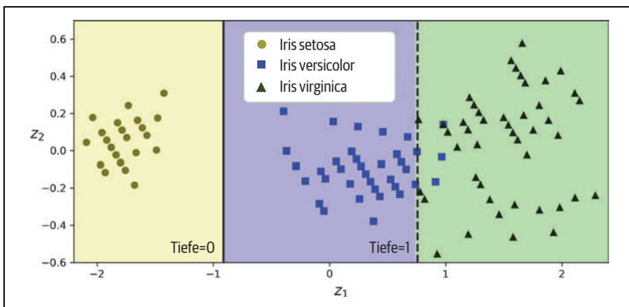
Abbildung 6-8: Die Entscheidungsgrenzen eines Baums mit dem skalierten und per PCA rotierten Iris-Datensatz
