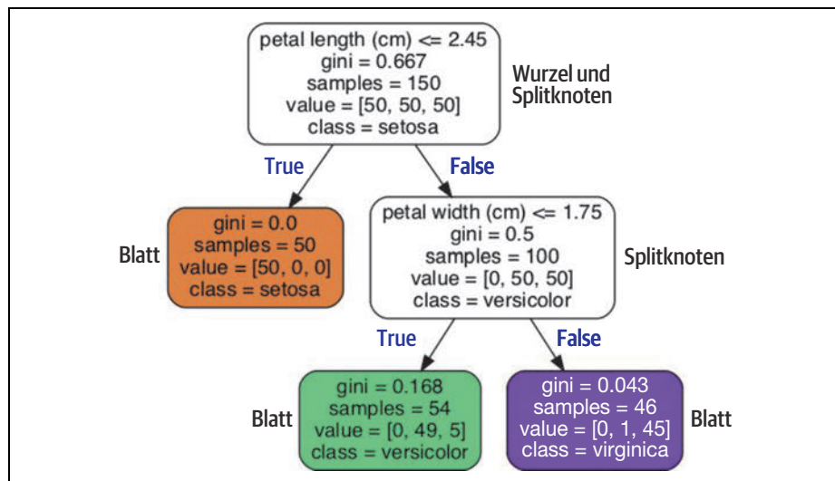
Abbildung 6-1: Iris-Entscheidungsbaum
