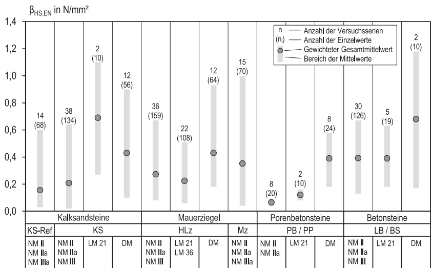
Bild 4. Bandbreite der Haftscherfestigkeitswerte nach dem EN-Verfahren (Werte aus [7])
