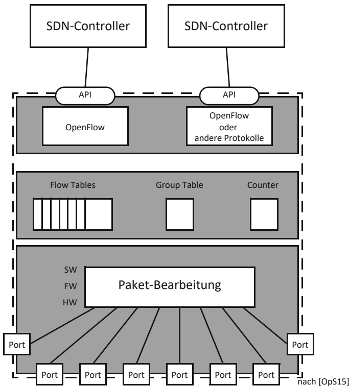
Abb. 223: Aufbau eines SDN-Netzelements
