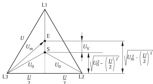
Bild 5.17 Spannung des Sternpunkts gegen Erde bei Erdschluss des Außenleiters L1
