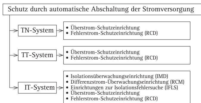
Bild 5.2 Schutzeinrichtungen für den „Schutz durch automatische Abschaltung der Stromversorgung“ in den verschiedenen Netzsystemen Hinweis: Zur RCM, IMD, IFLS und RCD siehe die diesbezüglichen Ausführungen im Kapitel 5.4
