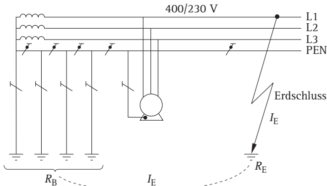
Bild 5.14 Erdschluss in einem Drehstromnetz 400/230 V
