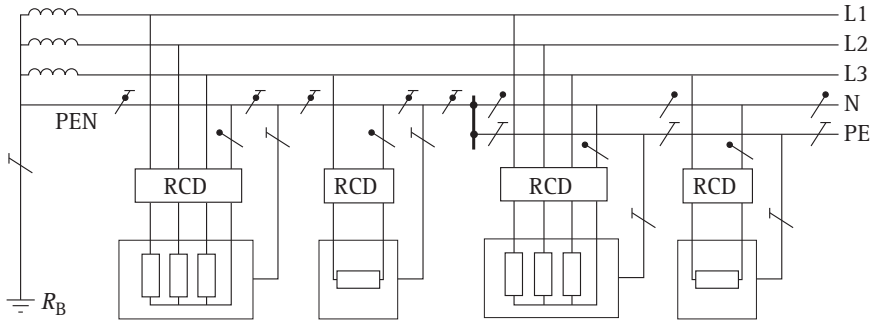
Bild 5.10 TN-System mit RCDs
