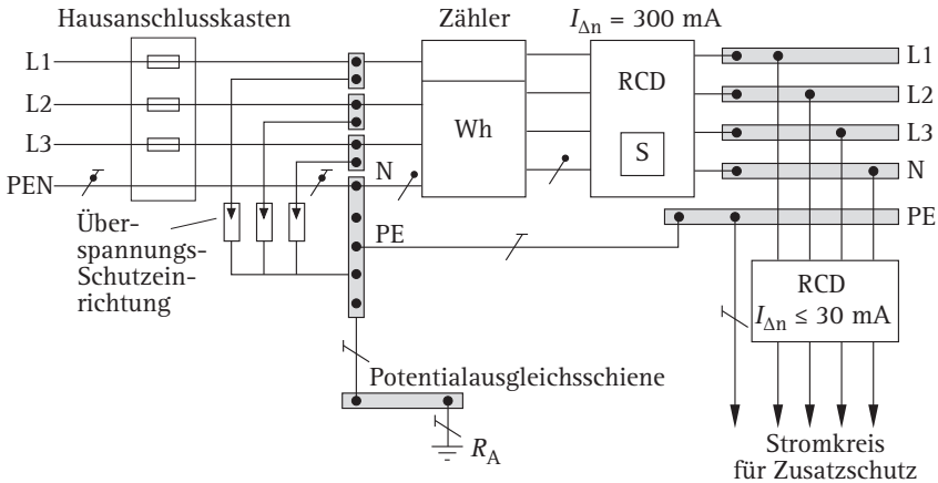
Bild 5.11 Schutzsystem, bestehend aus Überstrom-Schutzeinrichtungen, Überspannungsschutzeinrichtung und zwei Fehlerstrom-Schutzeinrichtungen (RCDs), um den Schutz durch automatische Abschaltung der Stromversorgung, den zusätzlichen Schutz, Belange des Brandschutzes sowie des Überspannungsschutzes zu gewährleisten
