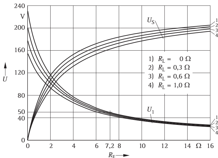
Bild 5.16 Spannungsverteilung an R_B und R_E
