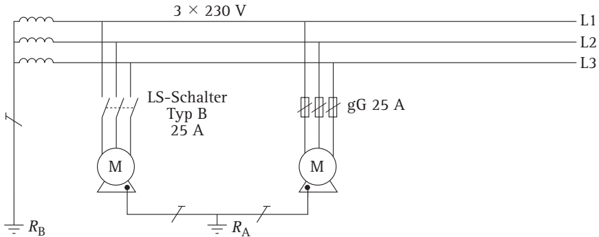
Bild 5.21 Beispiel für Abschaltung im TT-System
