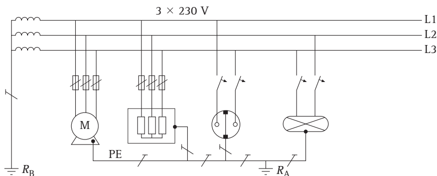
Bild 5.20 TT-System mit Überstrom-Schutzeinrichtungen
