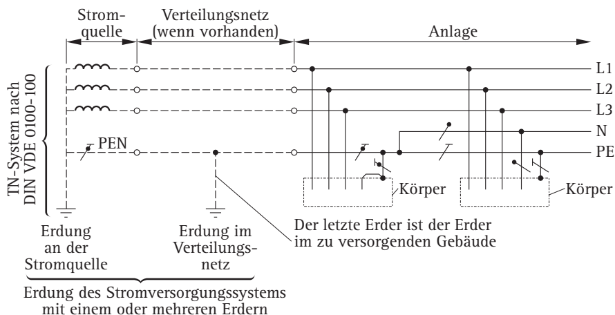
Bild 5.12 Darstellung eines TN-C-S-Systems nach DIN VDE 0100-100
