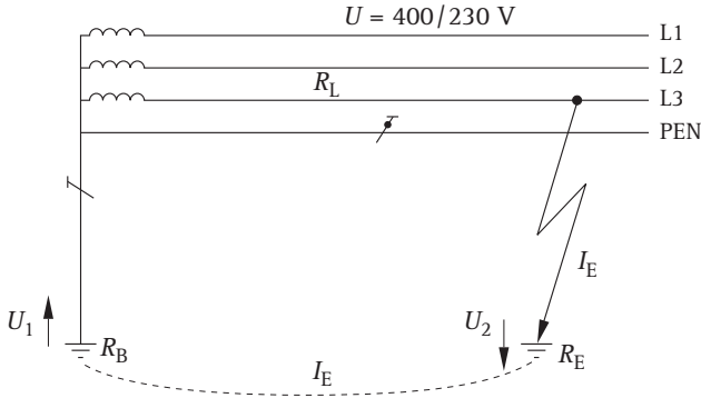
Bild 5.15 Verhältnis von R_B/R_E
