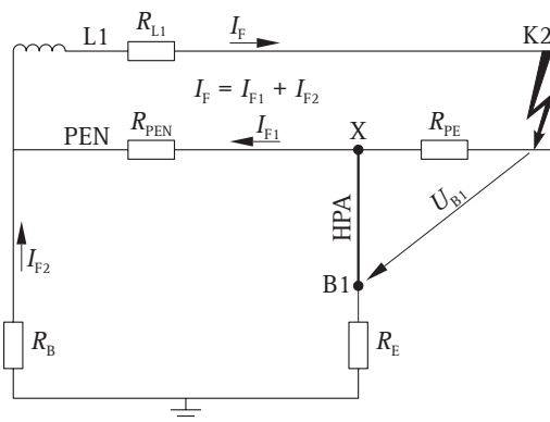
Bild 5.5 Ersatzschaltbild der Situation bei einem Isolationsfehler bei K2 nach Bild 5.3. Die berührbare Fehlerspannung U_{B1} reduziert sich um den Betrag, den der Fehlerstrom zwischen Punkt X und dem Sternpunkt des Transformators verursacht. U_{B1} entspricht somit im Wesentlichen dem Spannungsfall, den der Fehlerstrom I_F über den Schutzleiter PE im Gebäude verursacht.
