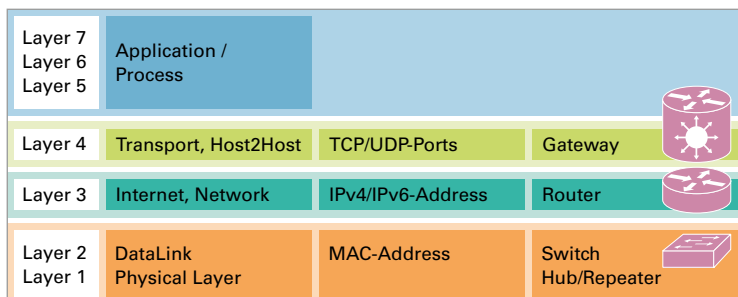
Bild 1.6: Adressen und Geräte im Netzwerk
