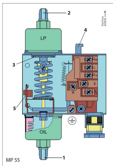
Abb. 10.9: Aufbau des Öldruckdifferenzschalters MP55 (Quelle: Danfoss)
