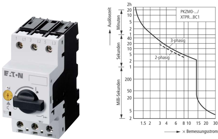
Abb. 10.5: Motorschutzschalter PKZM und Auslösekennlinie (Quelle: Eaton)
