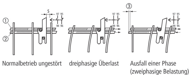
Abb. 10.1: Phasenempfindlichkeit mithilfe einer Auslöse- und Differenzialbrücke (Quelle: Eaton)
