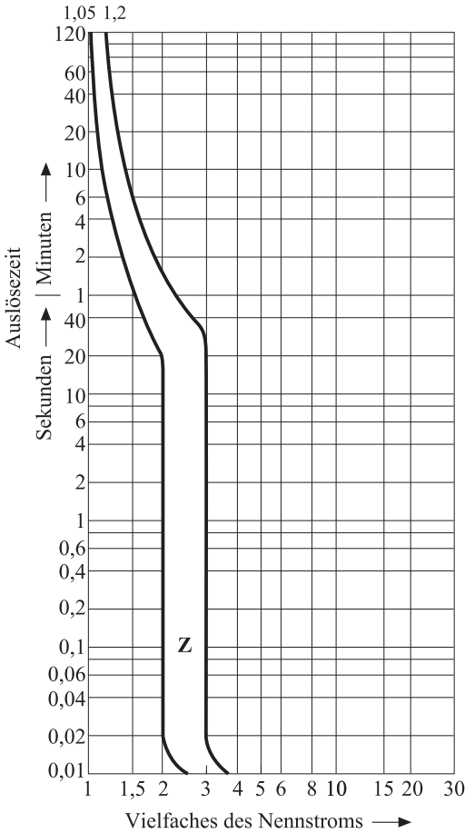
Bild 6.13 Leitungsschutzschalter – Charakteristik Z
