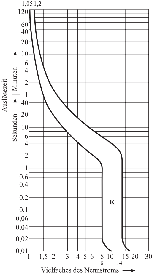
Bild 6.11 Leitungsschutzschalter – Charakteristik K
