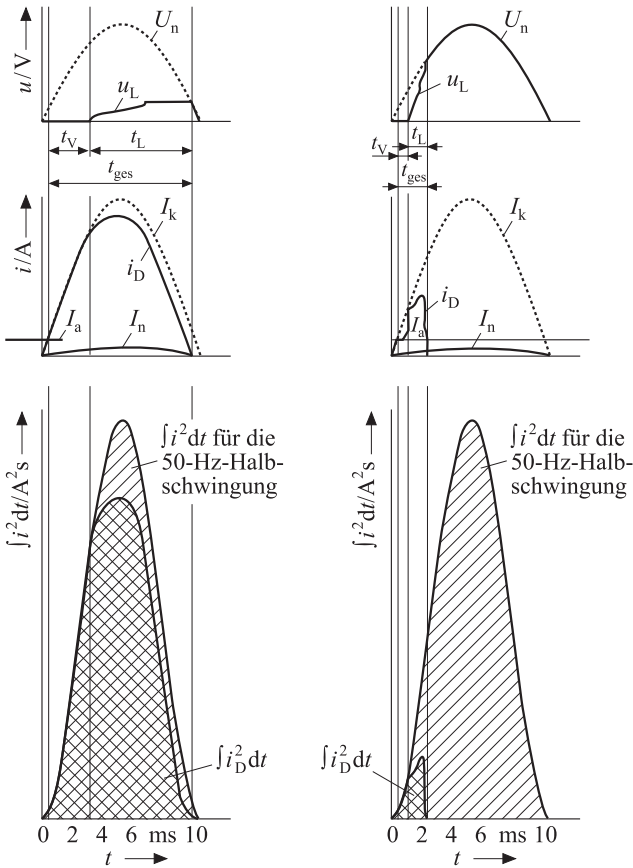
Bild 6.5 Abhängigkeit des Durchlassstroms i_D vom Durchlasswert I^2 \cdot t
