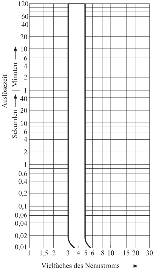
Bild 6.4 Verlauf der Auslösekennlinie des Elektromagnetauslösers eines Leitungsschutzschalters
