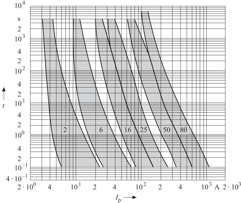
Bild 6.2a Zeit–Strom-Bereiche für „gG“-Sicherungseinsätze (Quelle: DIN VDE 0636-3:2024-01, Bild 101)
