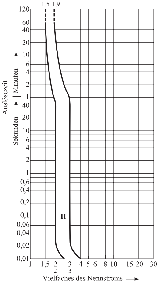
Bild 6.9 Leitungsschutzschalter – Charakteristik H
