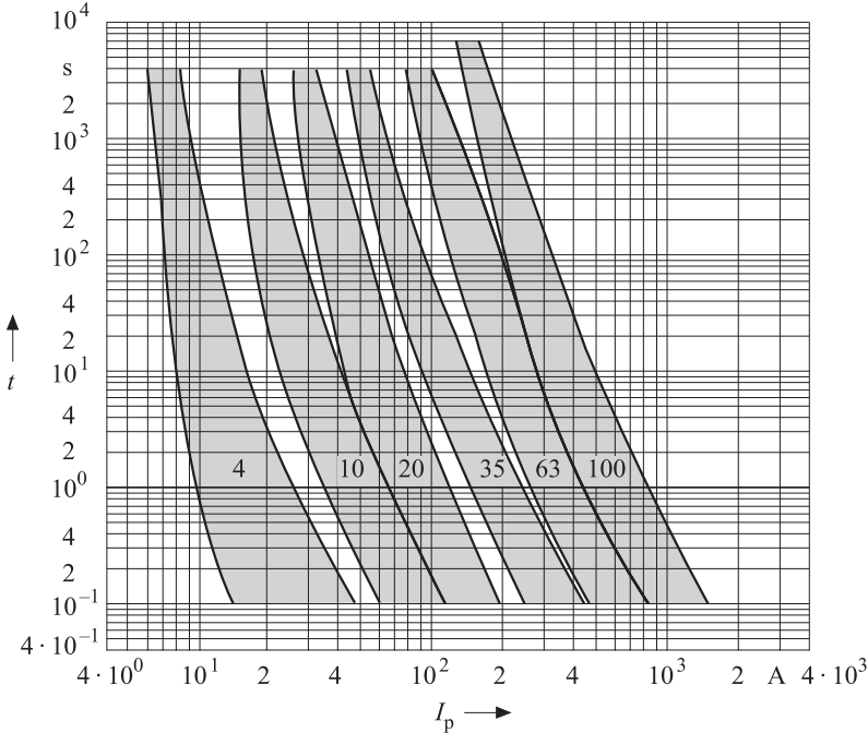
Bild 6.2b Zeit–Strom-Bereiche für „gG“-Sicherungseinsätze (Quelle: DIN VDE 0636-3:2024-01, Bild 102)
