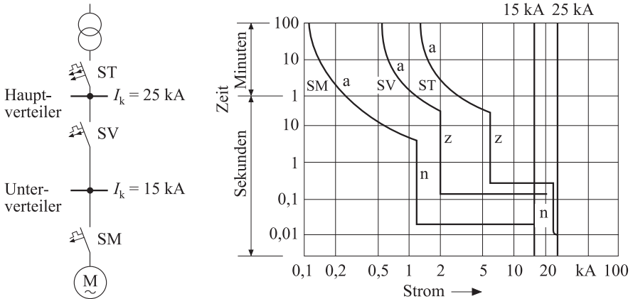
Bild 6.16 Auslösekennlinien von drei zueinander selektiv eingestellten Leistungsschaltern
