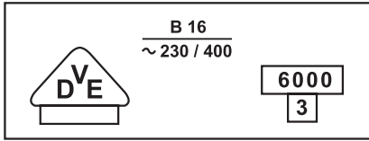
Bild 6.15 Aufschriften auf einem Leitungsschutzschalter
