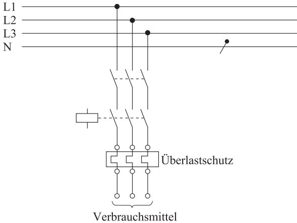
Bild 6.17 Schutz bei Überlast durch Schütz mit Überstromauslöser
