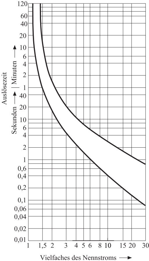
Bild 6.3 Verlauf der Auslösekennlinie des Thermo-Bimetallauslösers eines Leitungsschutzschalters
