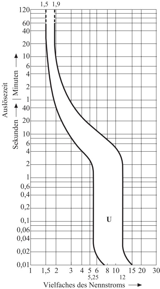
Bild 6.12 Leitungsschutzschalter – Charakteristik U
