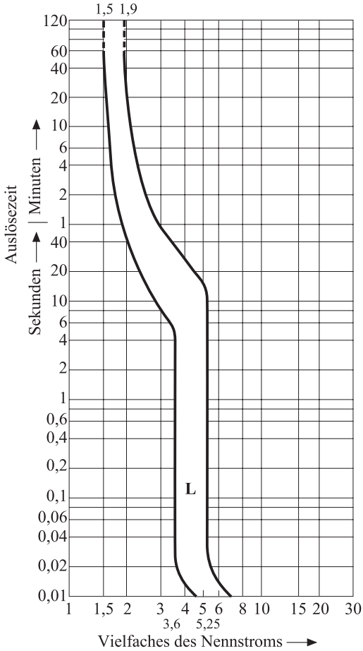
Bild 6.8 Leitungsschutzschalter – Charakteristik L
