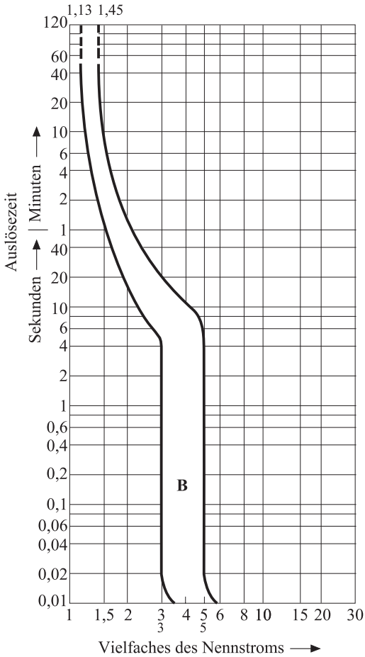
Bild 6.6 Leitungsschutzschalter – Charakteristik B
