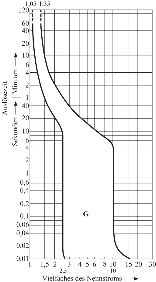
Bild 6.10 Leitungsschutzschalter – Charakteristik G
