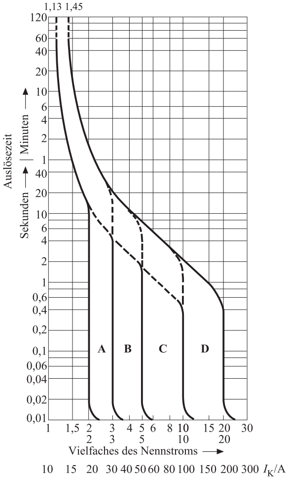
Bild 6.14 Leitungsschutzschalter – Auslösecharakteristiken A, B, C und D
