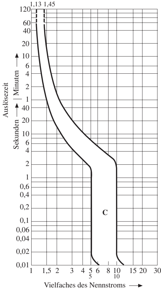
Bild 6.7 Leitungsschutzschalter – Charakteristik C
