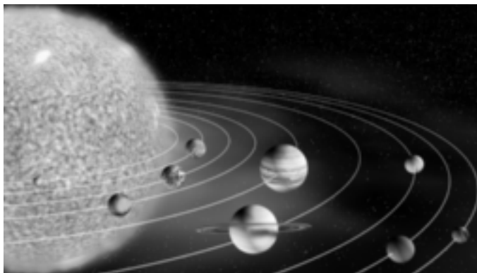
Abbildung 1: Das Sonnensystem
