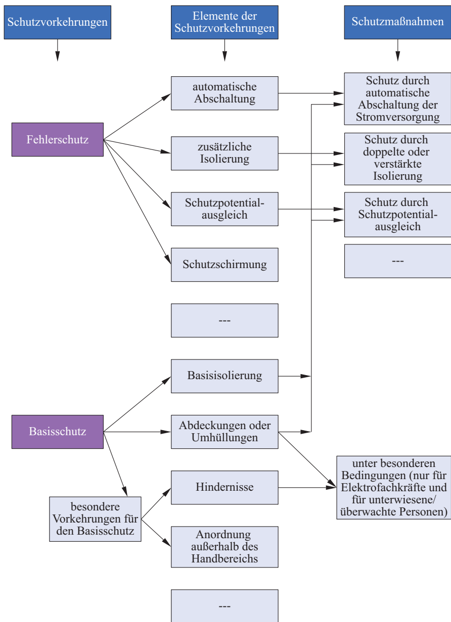
Bild 410-2 Beispiele von Schutzvorkehrungen und die daraus resultierenden Schutzmaßnahmen
