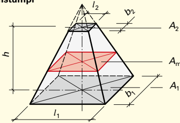
Pyramidenstumpf
