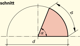
Kreisausschnitt
